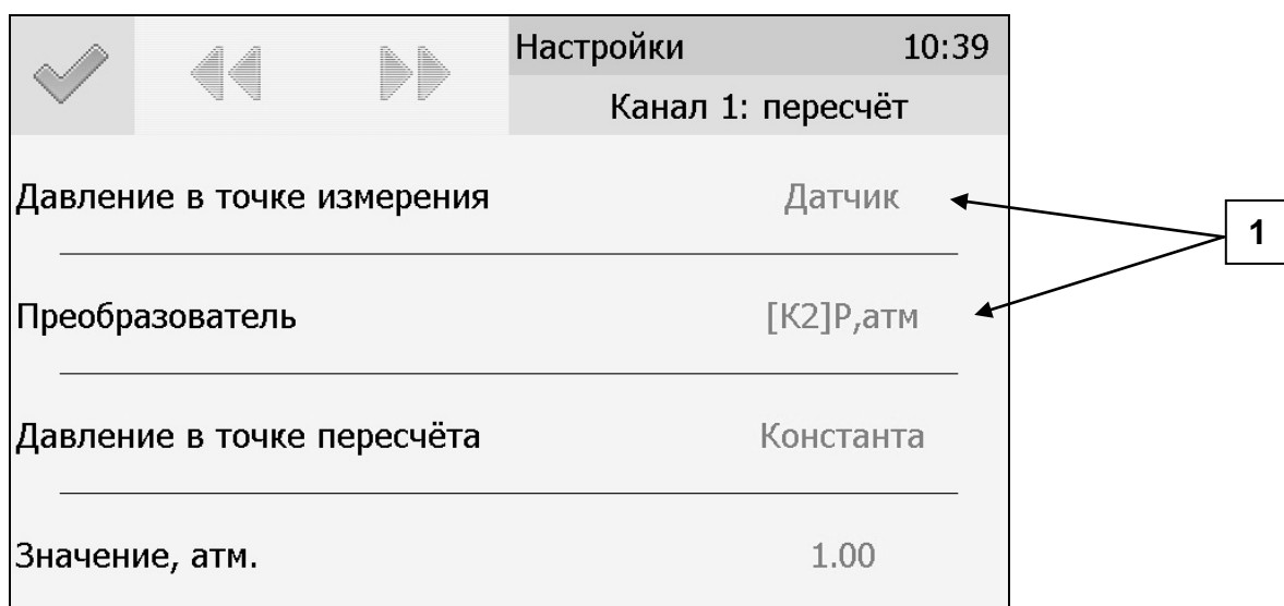
Рисунок 6.13 Настройка параметров пересчета влажности.
