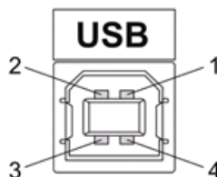
Рисунок 3.9 Разъем USB (розетка «B»)
