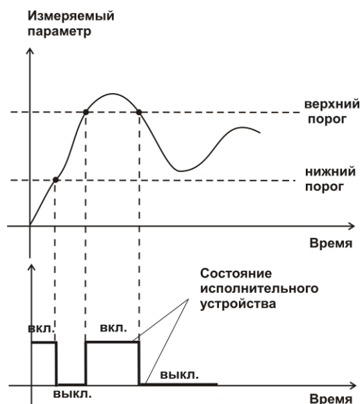
Рисунок 3.15 Функция вида f = НП+ВП
