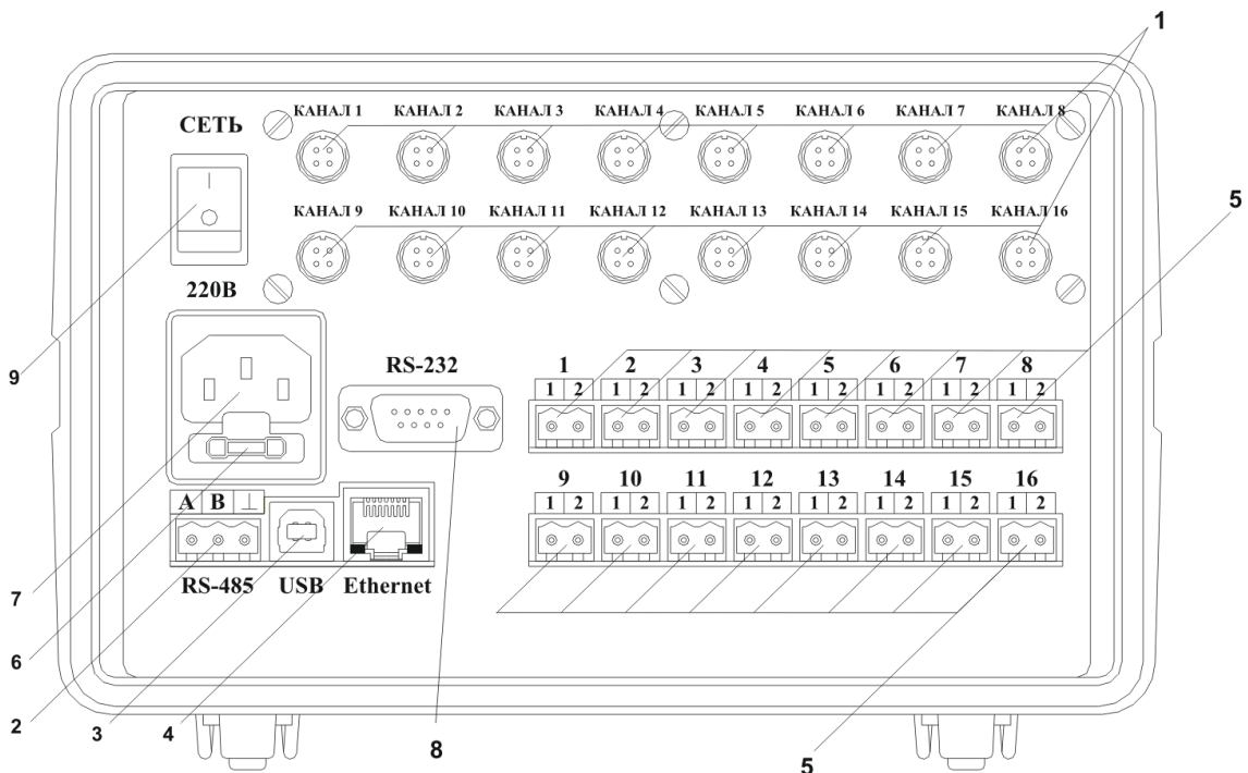
Рисунок 3.6 Вид задней панели приборов ИВГ-1 /8-Т-УР-ZА (7):
