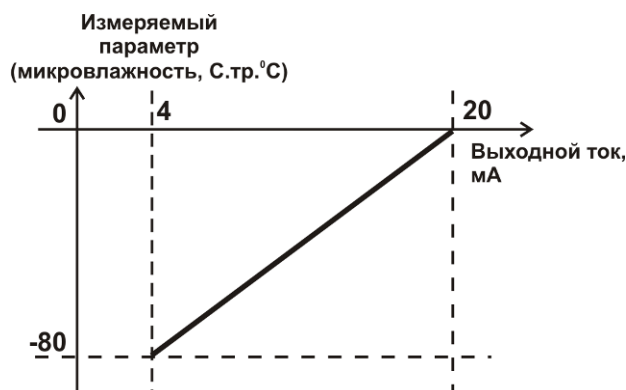
Рисунок 3.17 Линейный выход 4...20 мА по диапазону влажности -80...0 °С по точке росы
