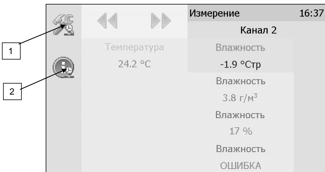
Рисунок 6.4 Вызов экрана настройки параметра.
