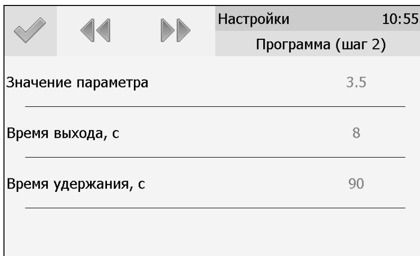
Рисунок 6.22 Вид экрана настройки второго шага программы регулирования
