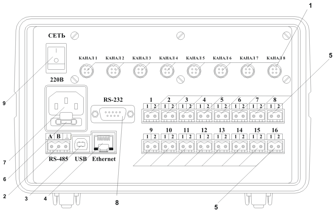
Рисунок 3.5 Вид задней панели приборов ИВГ-1 /4-Т-УР-ZА:
