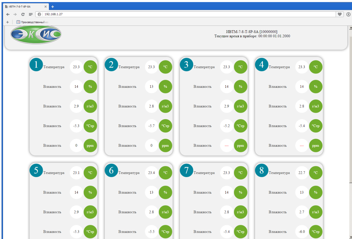
Рисунок 6.32 Web-интерфейс прибора ИВГ-1 /Х-Т-УР-ЗА.
