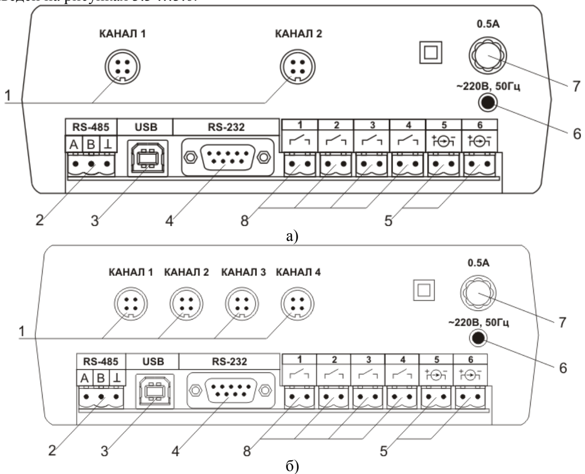
Рисунок 3.3 Вид задних панелей приборов ИВГ-1 /Х-Т-4Р-2А:
