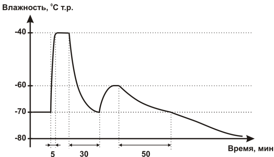
Рисунок 3.19 Время установления показаний при измерении точки росы газа
