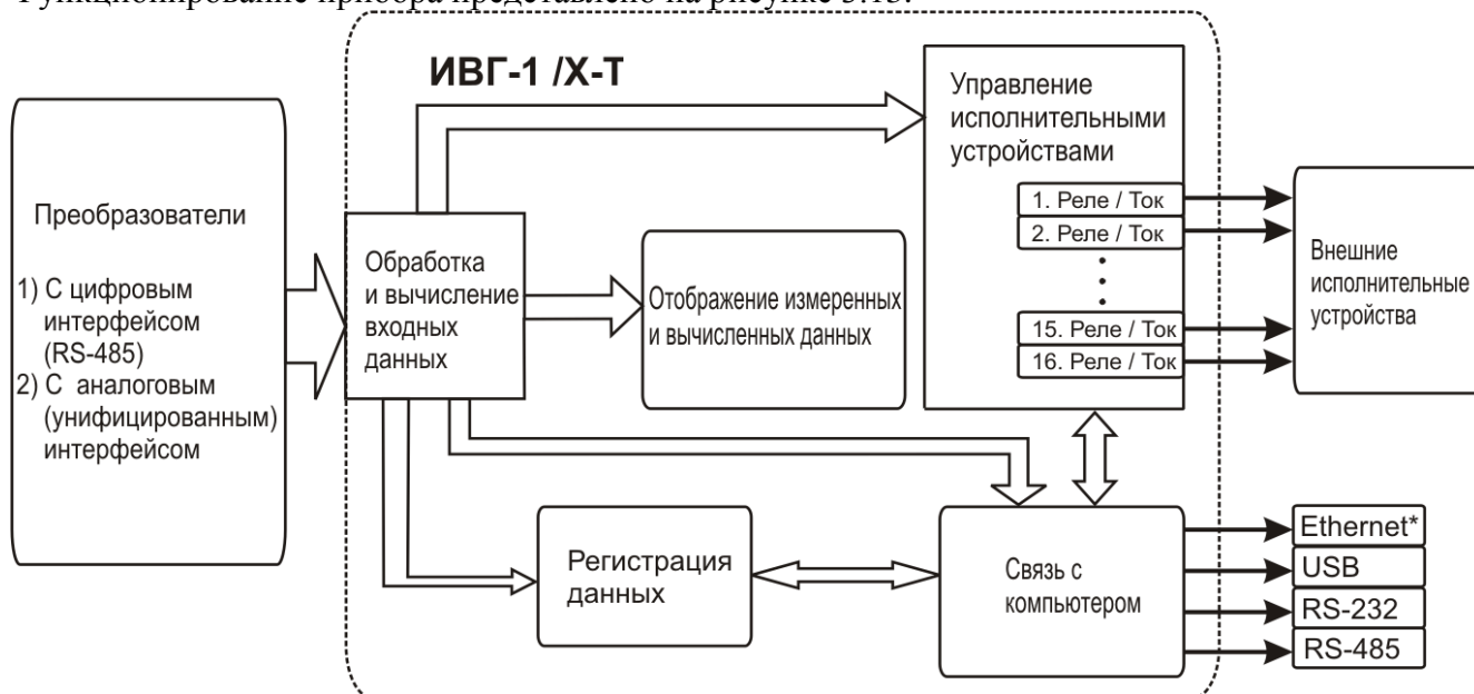
Рисунок 3.13 Функционирование прибора
