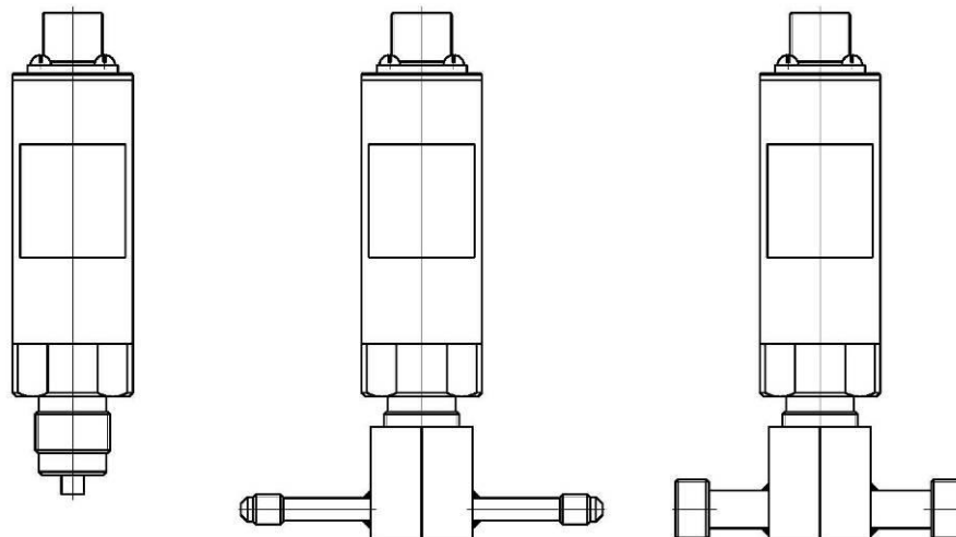
Рисунок 3.20 Измерительные преобразователи давления ИПД-02, ИПД-02-М8, ИПД-02-М16 (по порядку слева направо)
