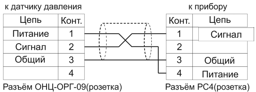
Разъём ОНЦ-ОРГ-09(розетка) со стороны монтажа
